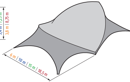
GESCHLOSSEN - BÖGEN OFFEN Überdachte Fläche 44 m 2 | 126 m 2 | 280 m 2 | 420 m 2
