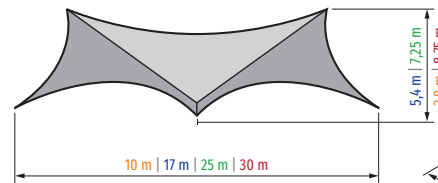
GESCHLOSSEN - BÖGEN OFFEN Überdachte Fläche 44 m 2 | 126 m 2 | 280 m 2 | 420 m 2
