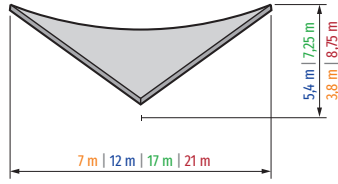
OFFEN Überdachte Fläche 32 m 2 | 90 m 2 | 190 m 2 | 286 m 2
