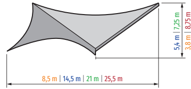
EINSEITIG GESCHLOSSEN - BÖGEN OFFEN Überdachte Fläche 38 m 2 | 108 m 2 | 235 m 2 | 353 m 2
