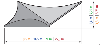
EINSEITIG GESCHLOSSEN - BÖGEN GESCHLOSSEN Überdachte Fläche 46 m 2 | 130 m 2 | 285 m 2 | 423 m 2
