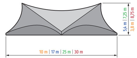
GESCHLOSSEN - BÖGEN GESCHLOSSEN Überdachte Fläche 60 m 2 | 170 m 2 | 380 m 2 | 560 m 2
