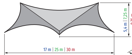
GESCHLOSSEN - BÖGEN OFFEN Überdachte Fläche 126 m 2 | 280 m 2 | 420 m 2
