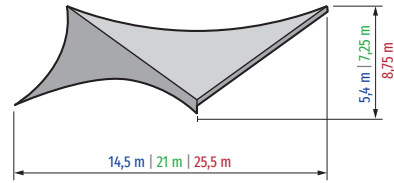
EINSEITIG GESCHLOSSEN - BÖGEN OFFEN Überdachte Fläche 108 m 2 | 235 m 2 | 353 m 2
