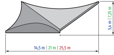
EINSEITIG GESCHLOSSEN - BÖGEN GESCHLOSSEN Überdachte Fläche 130 m 2 | 285 m 2 | 423 m 2
