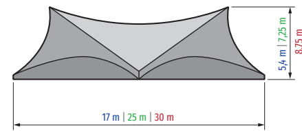
GESCHLOSSEN - BÖGEN GESCHLOSSEN Überdachte Fläche 170 m 2 | 380 m 2 | 560 m 2
